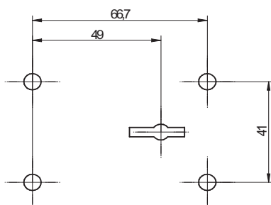
Abb. 3: Befestigungslochbild
