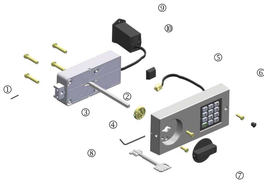
Abb. 4: Montageschritte
