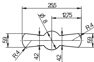
Abb. 1: Schlüsselführung 86101
