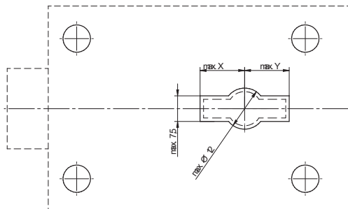
Abb. 2: Max. Lochquerschnitt
