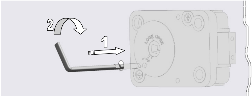
Abb. 2: Einführen Umstellschlüssel
