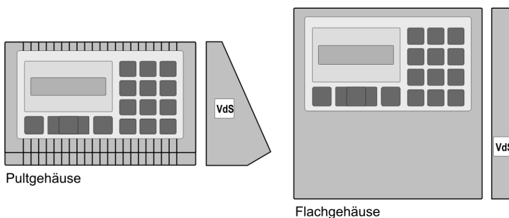
Abb. 5.18: Eingabeeinheit, Verplombung
