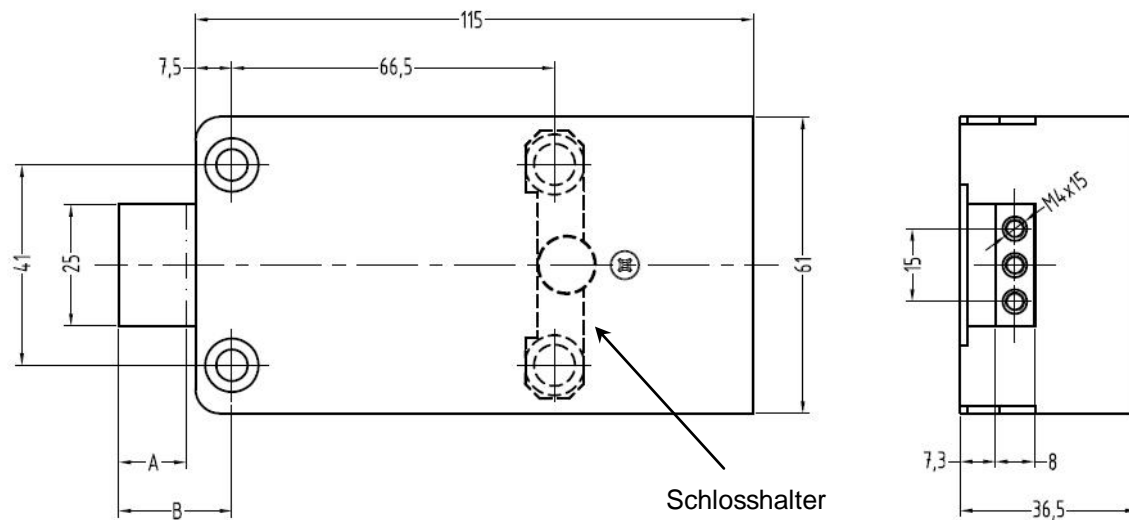
Abb. 5.8: Betätigung, Abmessungen
