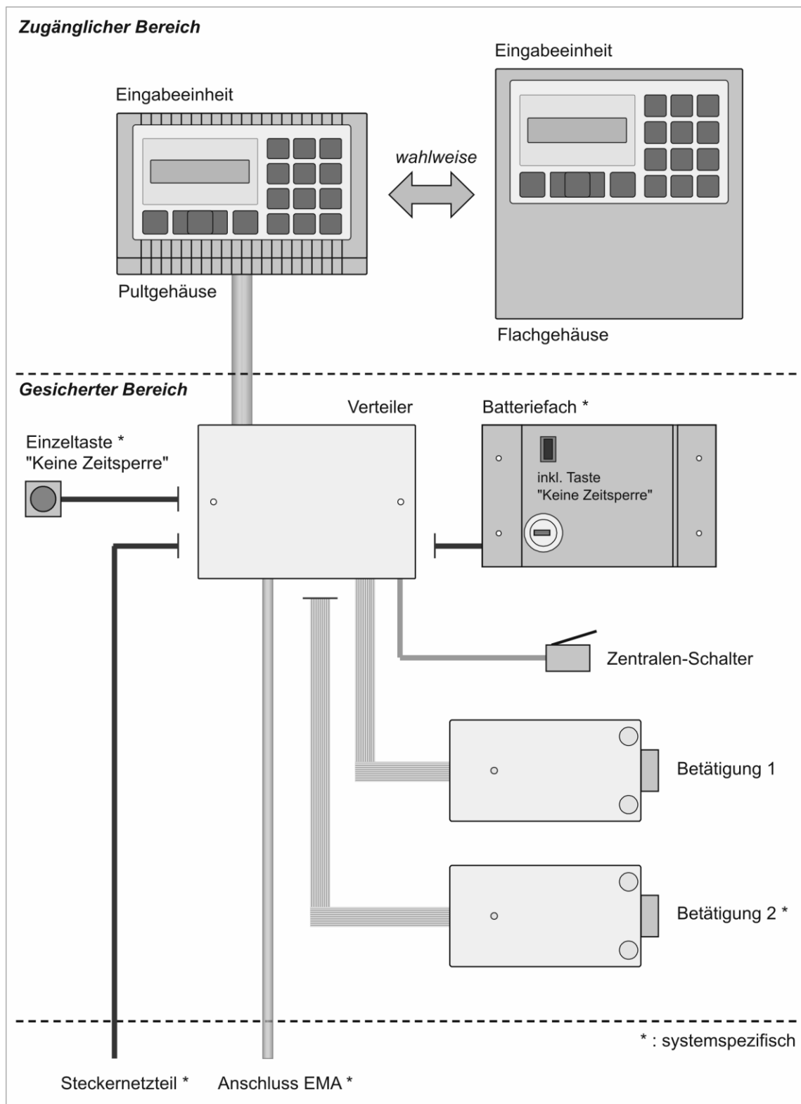
Abb. 3.1: Schlosssystem < SafeLock - one >, Übersicht
