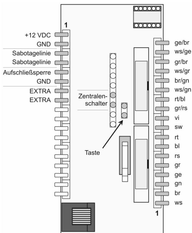
Abb. 5.13: Verteiler, Anschlussplan
