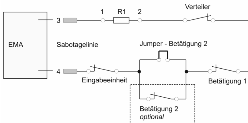
Abb. 5.15: EMA – Sabotagelinie, Anschlussplan
