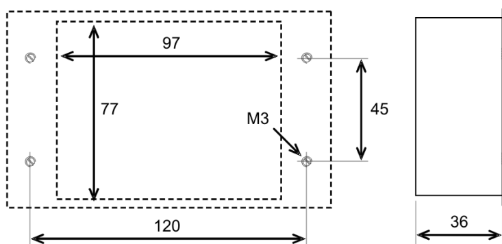
Abb. 5.10: Batteriefach, Bohrbild
