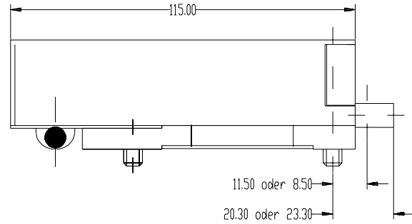
Betätigung Motorschloß
