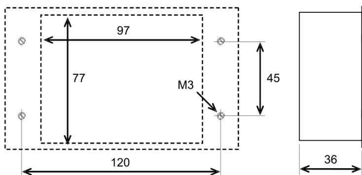
Abb. 6.10: Batteriefach, Bohrbild
