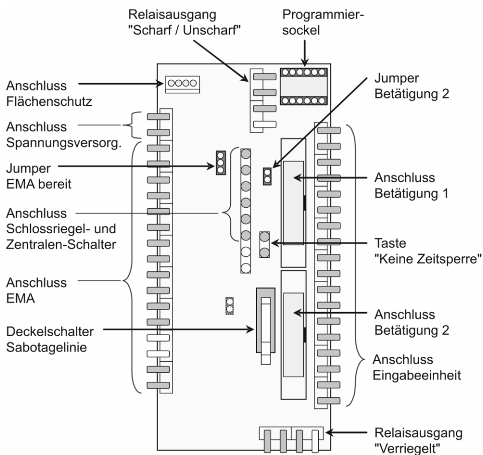
Abb. 6.18: Schalteinrichtung, Anschlussübersicht
