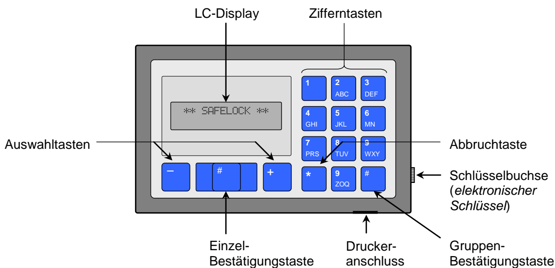
Abb. 3.1: Eingabeeinheit – Pultgehäuse, Vorderansicht
