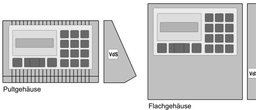
Abb. 6.27: Eingabeeinheit, Verplombung
