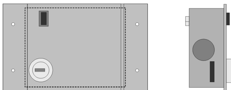
Abb. 6.11: Batteriefach, Detailansicht
