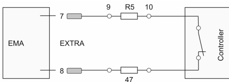
Abb. 6.17: EMA – EXTRA, Anschlussplan
