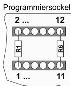
Abb. 6.21: Schalteinrichtung, Programmiersockel
