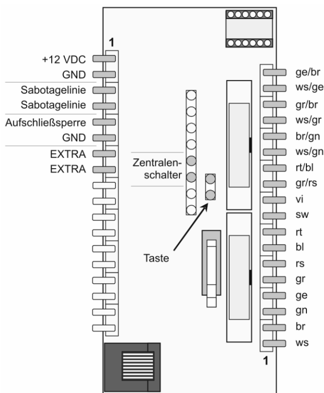
Abb. 6.13: Verteiler, Anschlussplan
