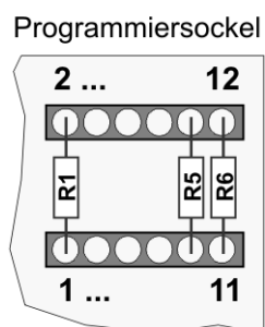
Abb. 6.14: Verteiler, Programmiersockel
