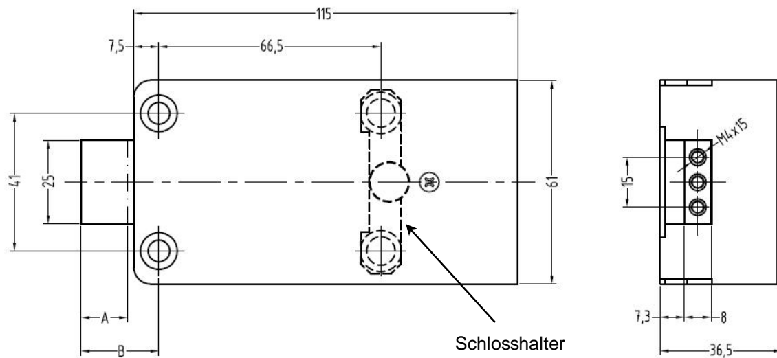
Abb. 6.8: Betätigung, Abmessungen
