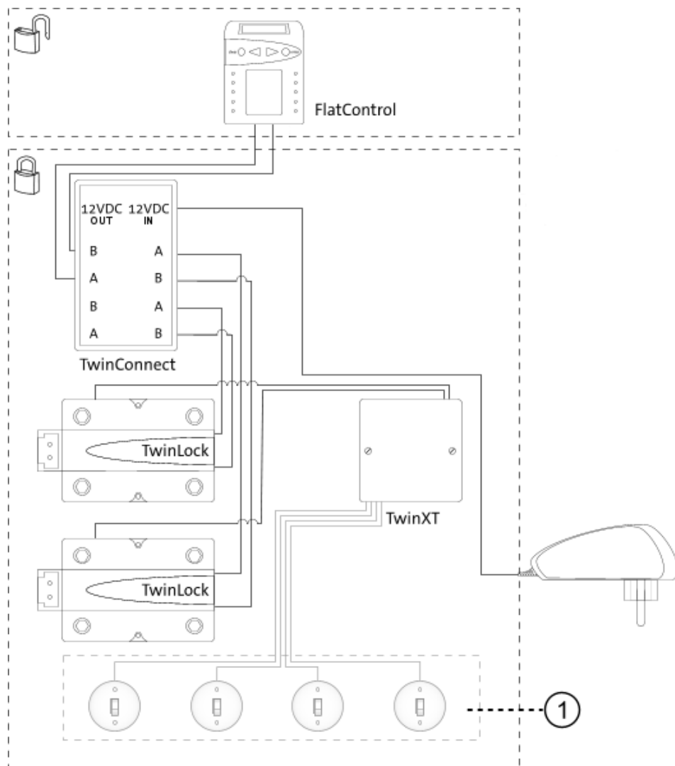
Abbildung 2 Systemaufbau von Basissystem 2.1
