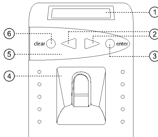
Abbildung 18 Bedieneinheit FlatControl BioPIN
