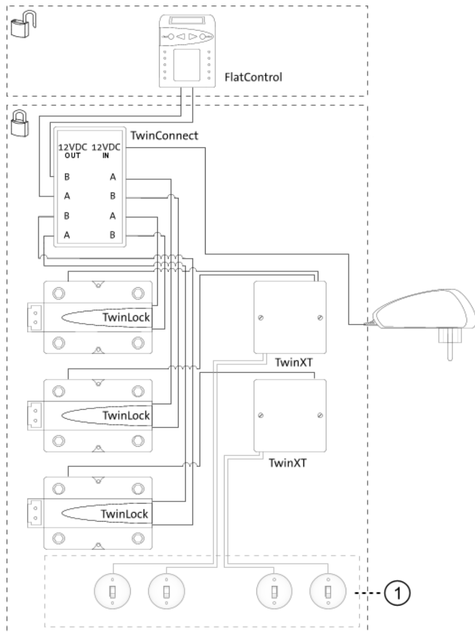
Abbildung 3 Systemaufbau von Basissystem 3.2
