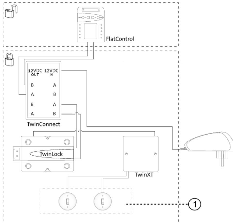
Abbildung 1 Systemaufbau von Basissystem 1.1
