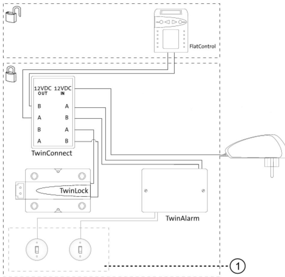
Abbildung 4 Systemaufbau von Komfortsystem 1 ohne EMA
